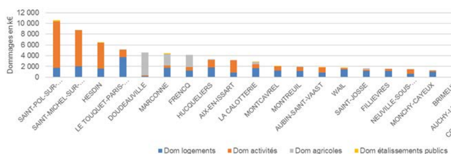
Figure 3-1 : Dommages par communes par enjeu pour un événement centennal
