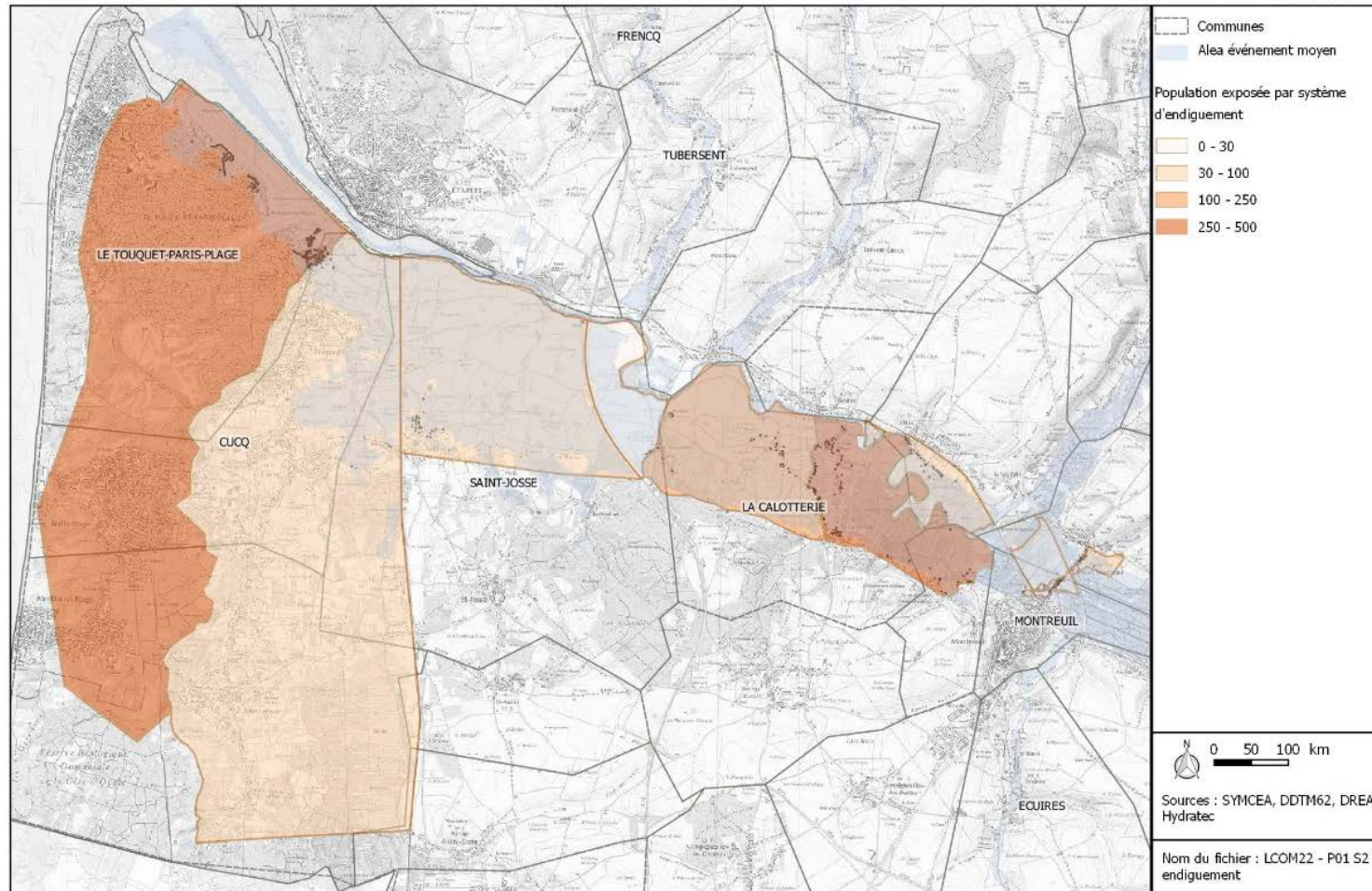
Figure 3-8 : Population exposée à un événement moyen, par système d'endiguement
