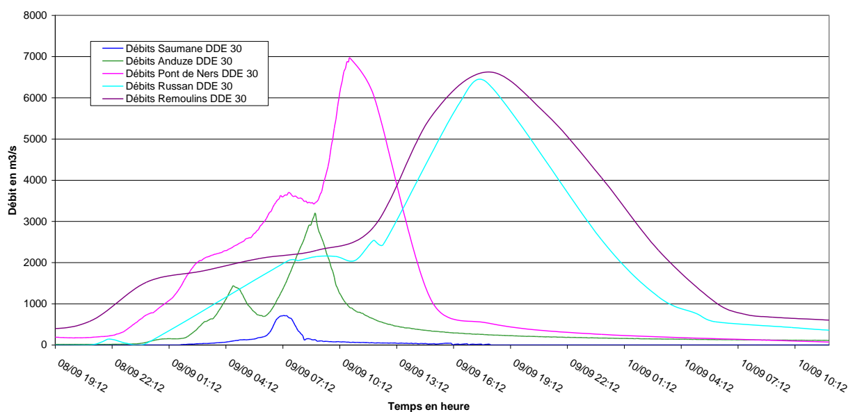
Figure 3 : Hydrogramme de la crue du 9 Septembre 2002 au droit des stations de suivi
