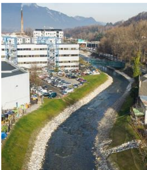
Augmentation de la section de la rivière dans un secteur inondable en février 1990. 2015.
