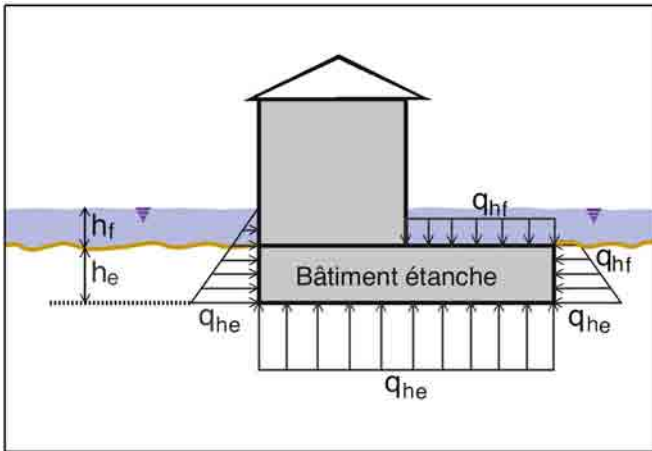
Figure 5.3 Crués : pression résultant de la contrainte hydrostatique (suivant VKF-AEAI)
